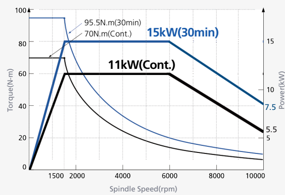
VESTA-610D
